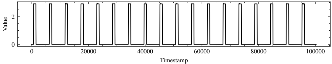
I_Load3
